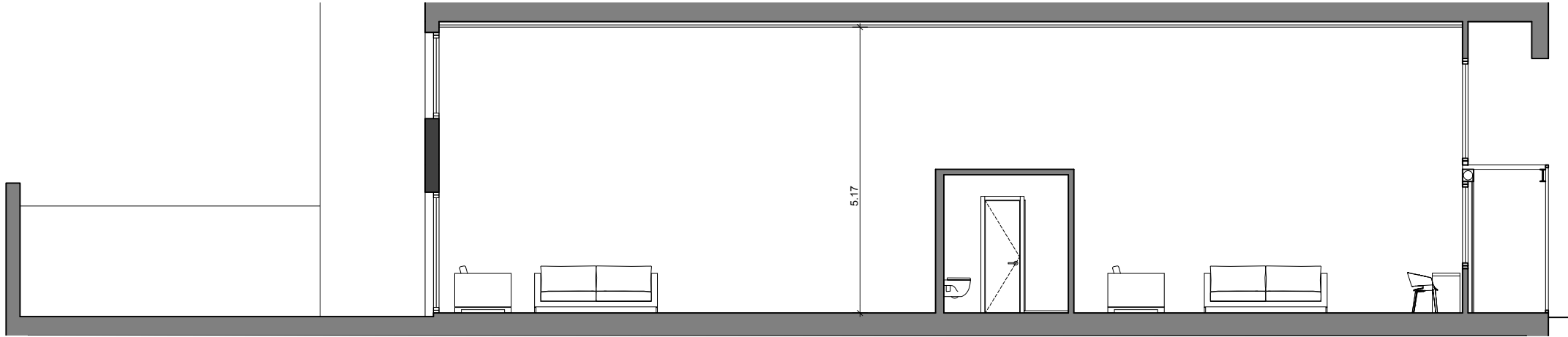
Sección longitudinal
