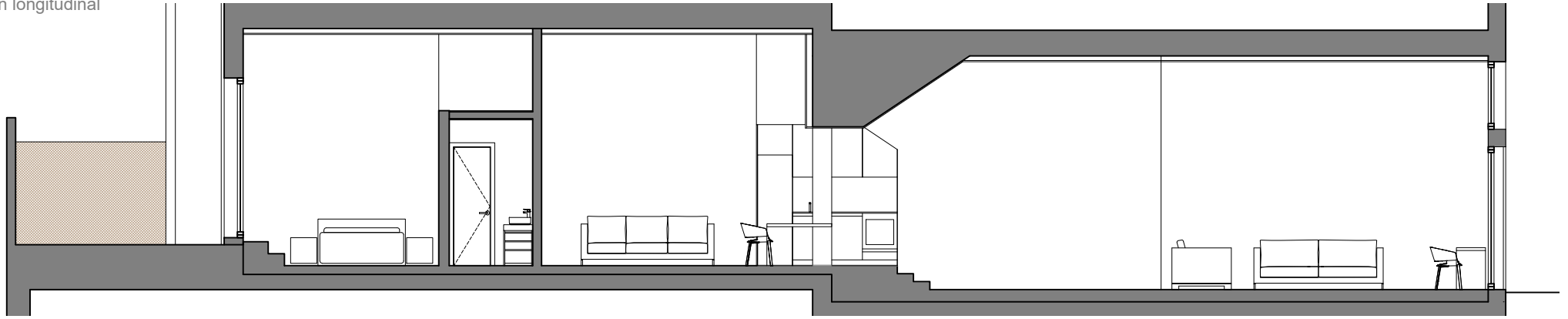
Sección longitudinal
