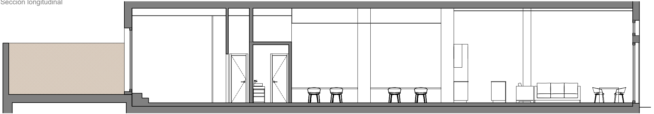
Sección longitudinal
